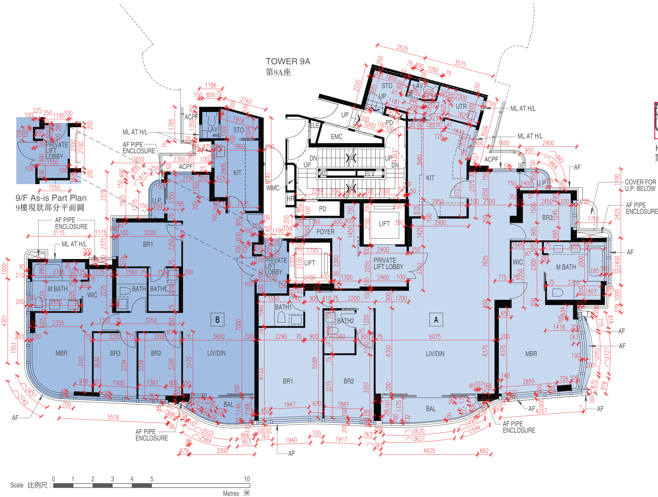
TOWER 9 9/F 第9座 9樓
