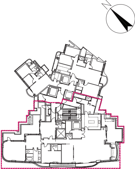
KEY PLAN FOR TOWER 9/9A 26/F 第9/9A座 26樓 位置圖
