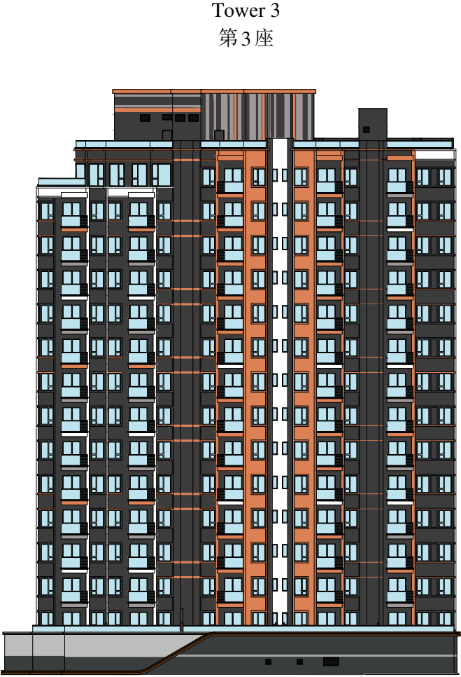
Elevation Plan 11 立面圖 11
