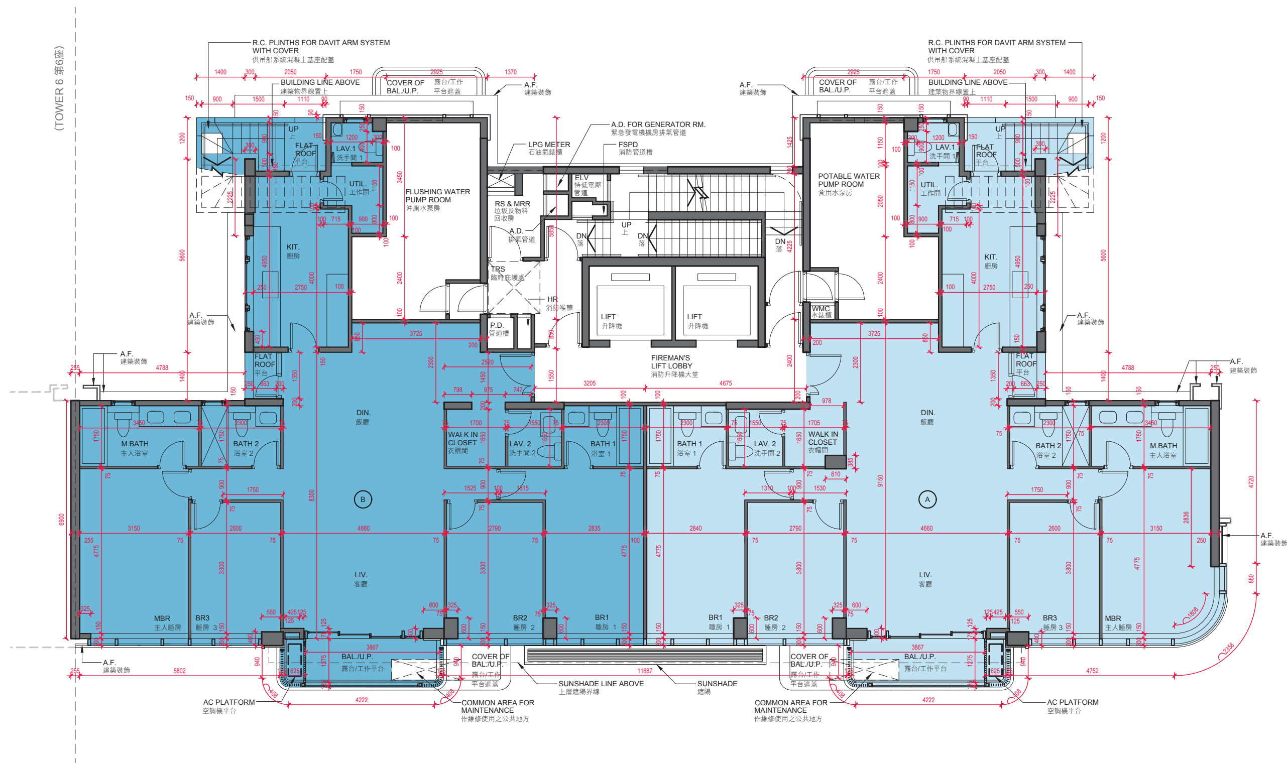
TOWER 3 16/F FLOOR PLAN 第3座 16樓樓面平面圖
